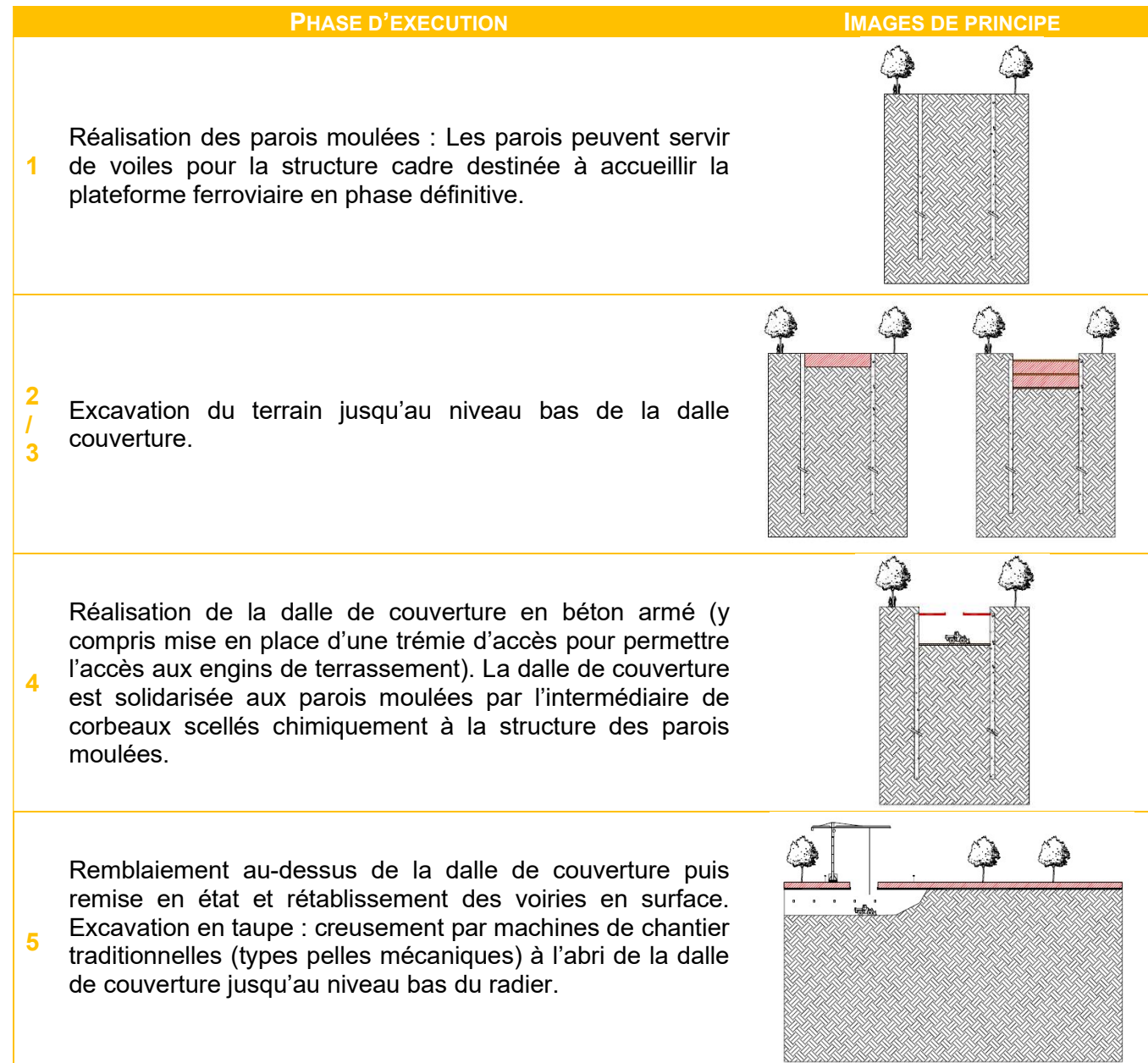
Figure 83 – Phasage de réalisation d'une excavation en tranchée couverte (Source : Ingérop)
