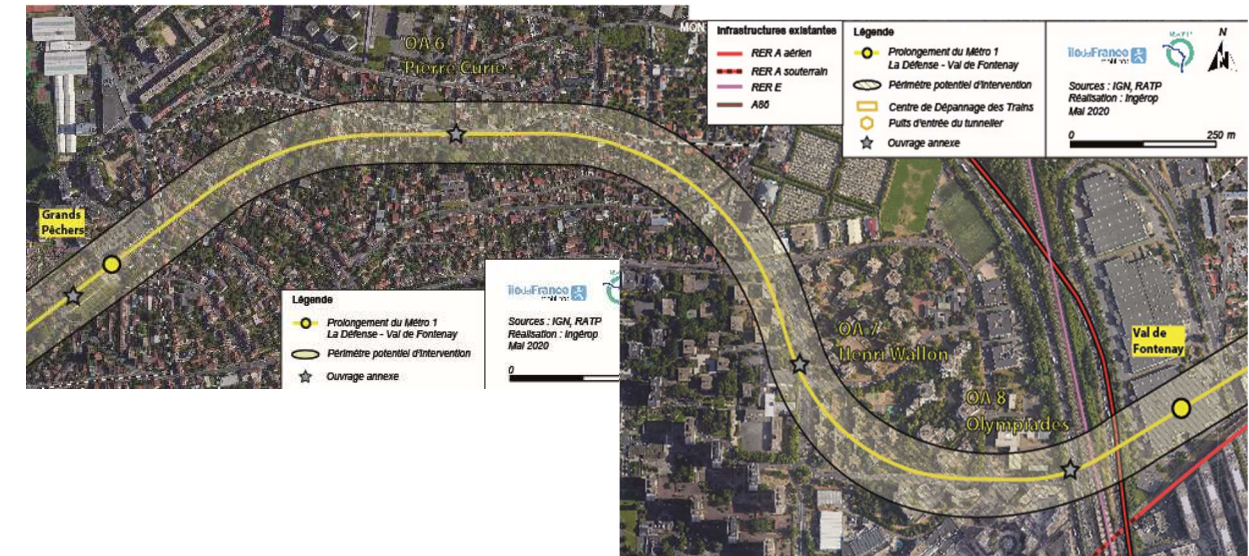
Figure 48 – Extrait du PGT – Zoom entre les stations Grands Pêchers et Val de Fontenay (Source : Ingérop)
