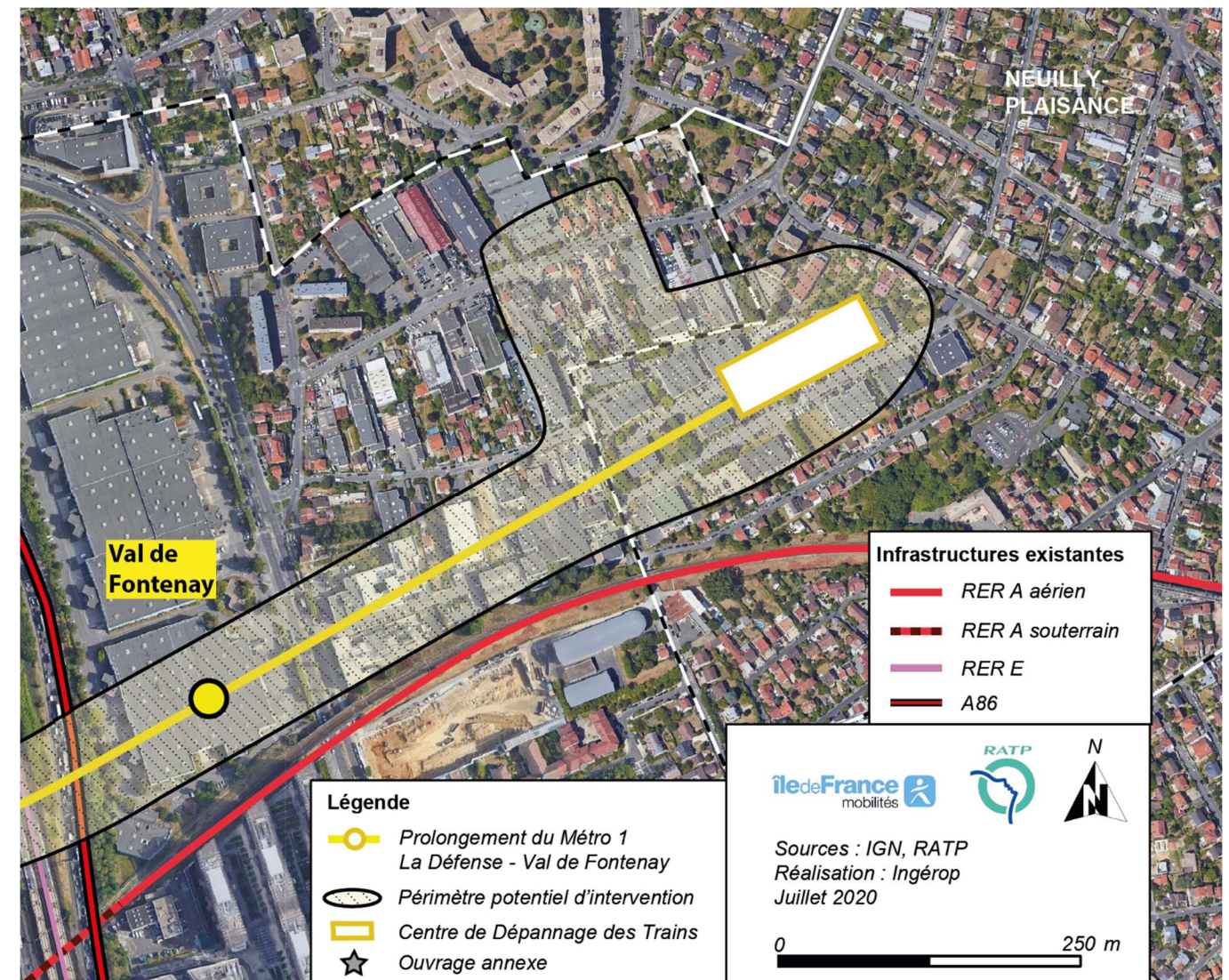
Figure 79 – Extrait du PGT – Zoom entre la station Val de Fontenay et le CDT (Source : Ingérop)
