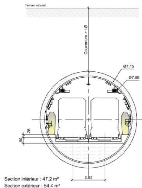
Figure 69 – Coupe-type du tunnel en section monotube
